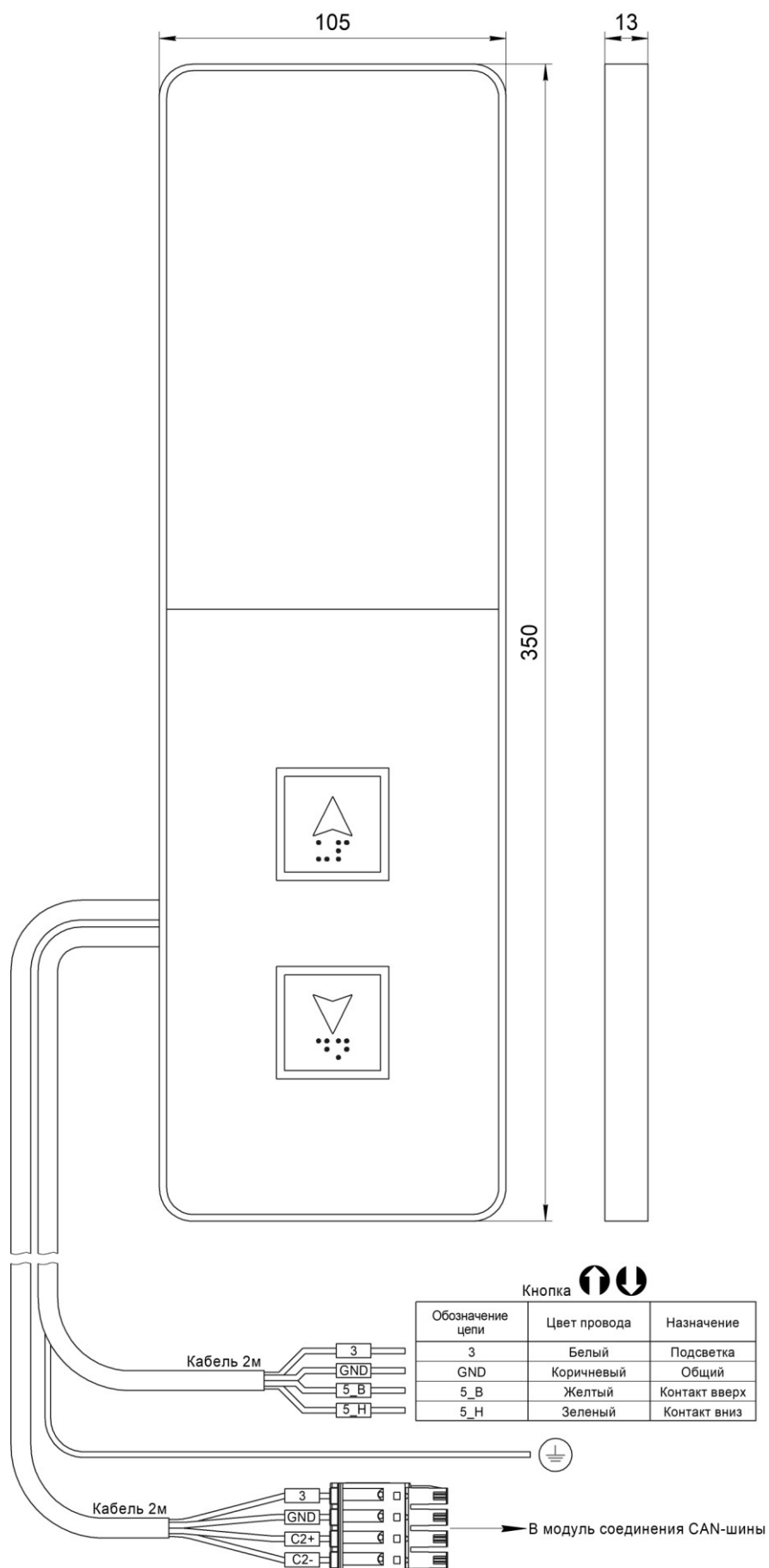
Рис.1 Внешний вид, габаритные и установочные размеры Вызывного поста МАЛАХИТ НШЕК.468381.087
